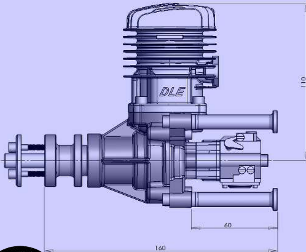
DLE35RA
